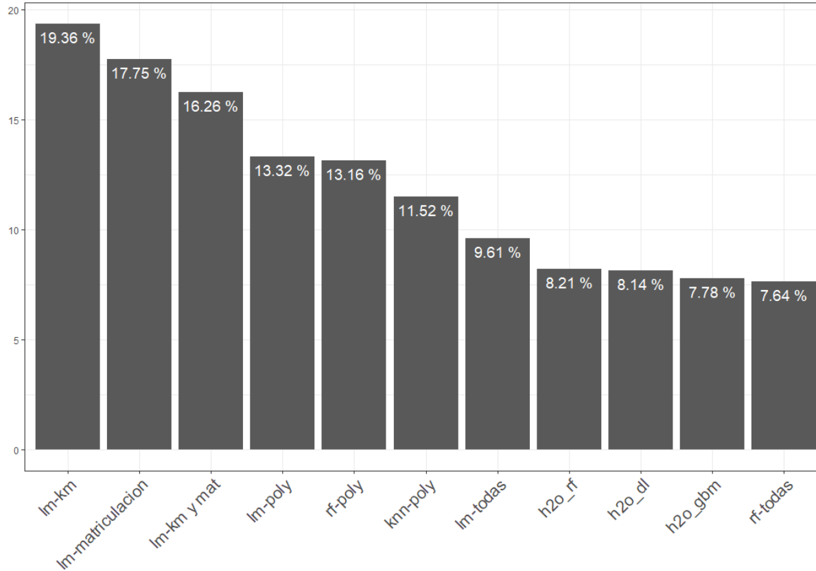
MAPE de los diferentes modelos
