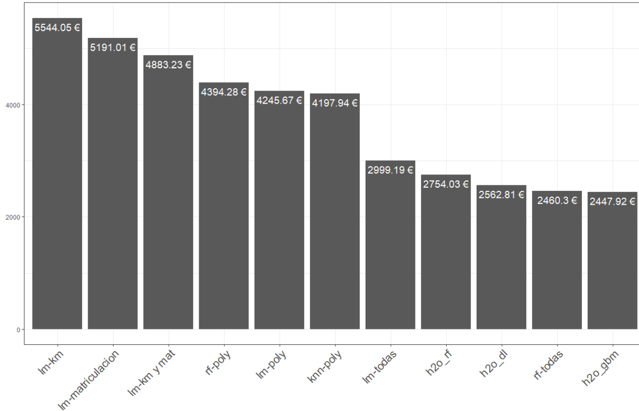
RMSE de los diferentes modelos
