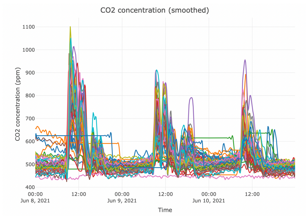
Figura 1. Evolución de la concentración de CO2 durante la ABAU.
