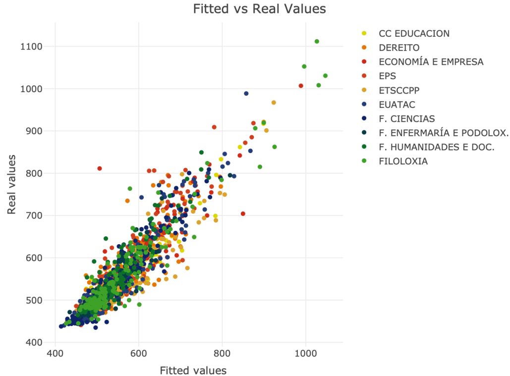
Figura 3. Valores reales frente a predichos.
