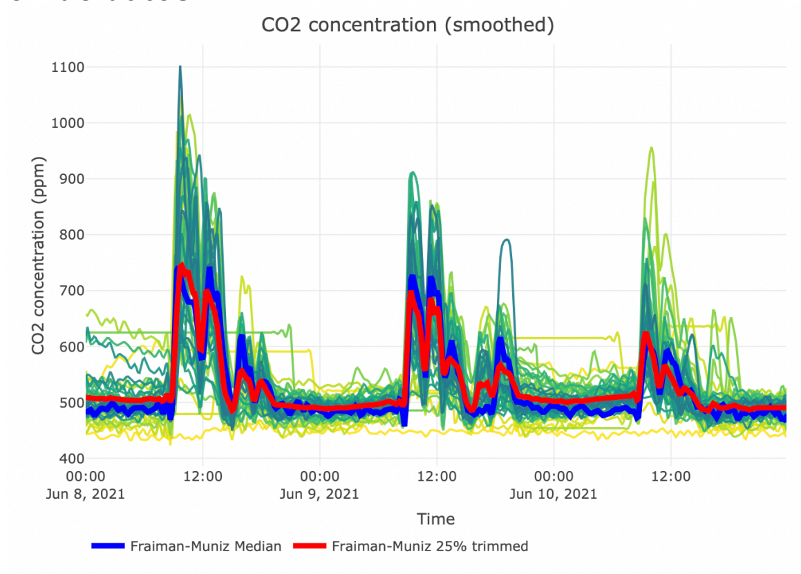
Figura 2. Profundidad de Fraiman-Muniz para las curvas de CO 2 .
